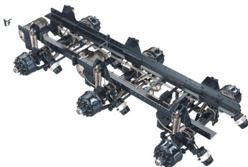
Train roulant avec châssis auxiliaire et gestion active de la suspension hydraulique
